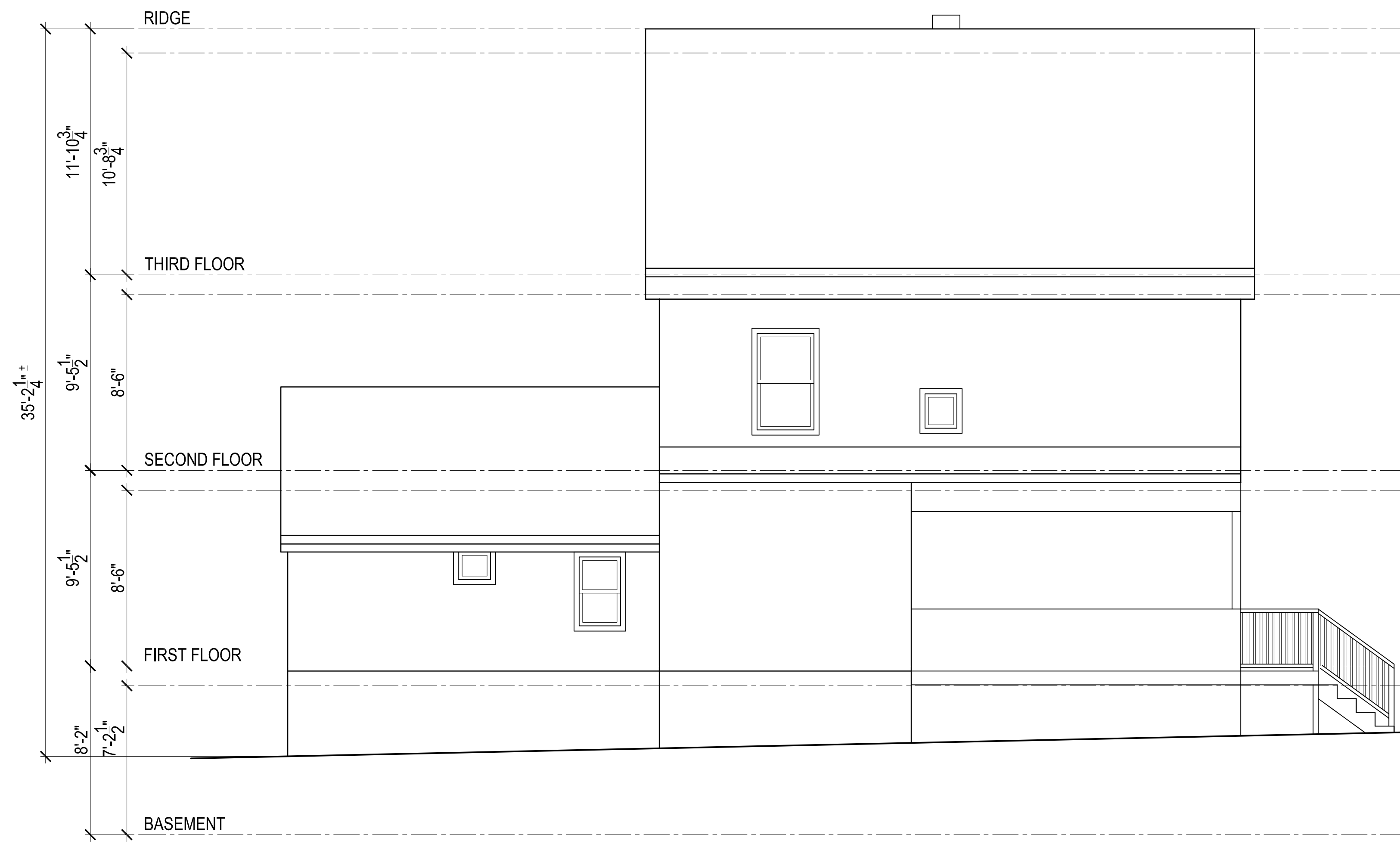
ELEVATION 4
